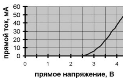
Зависимость прямого тока от прямого напряжения
