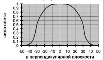
Диаграмма излучения - светодиоды с углом 30x60 градусов
